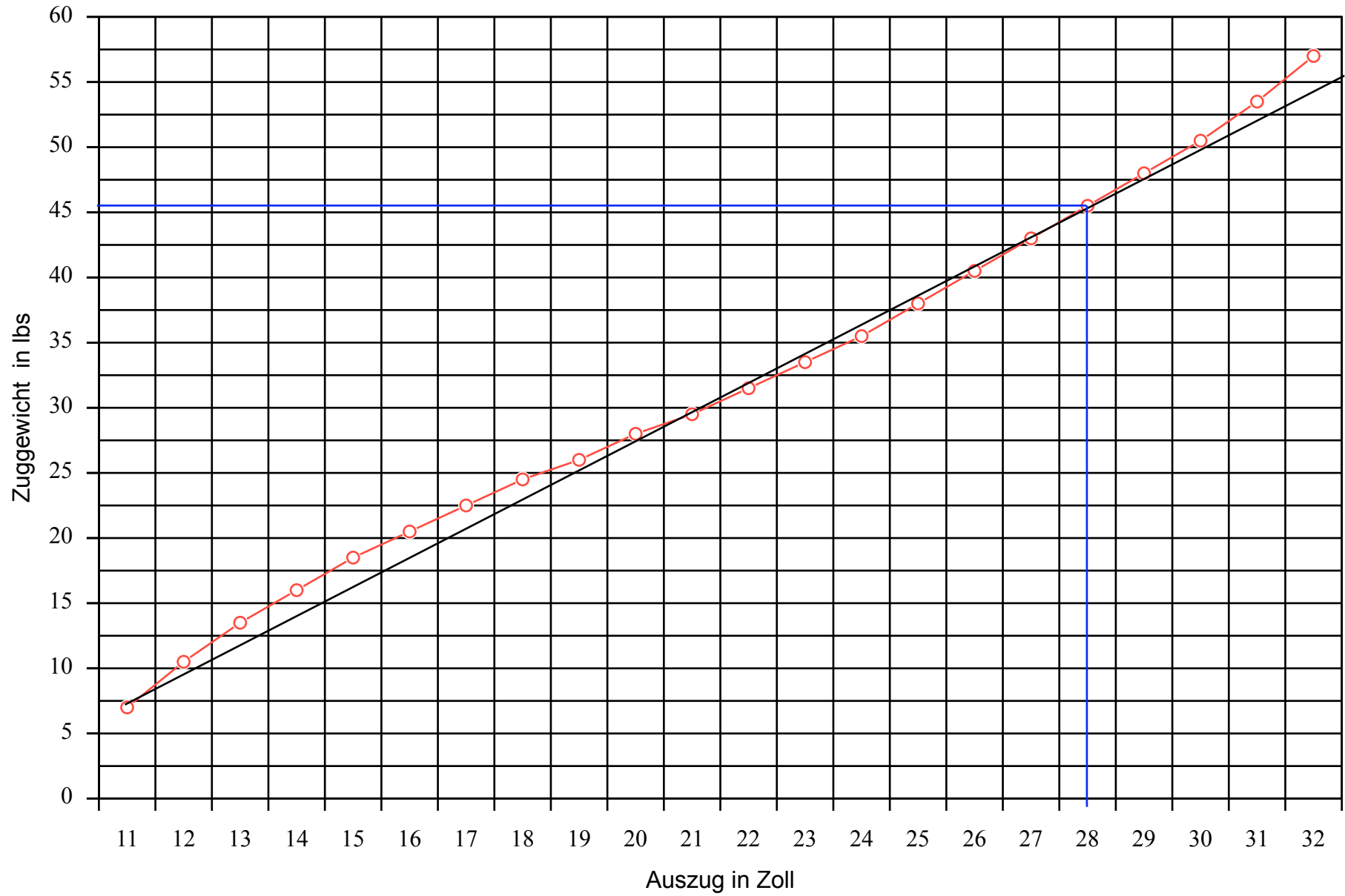
Auszugsdiagramm Bearpaw Serien Hawk 60", 45,5#/28"
