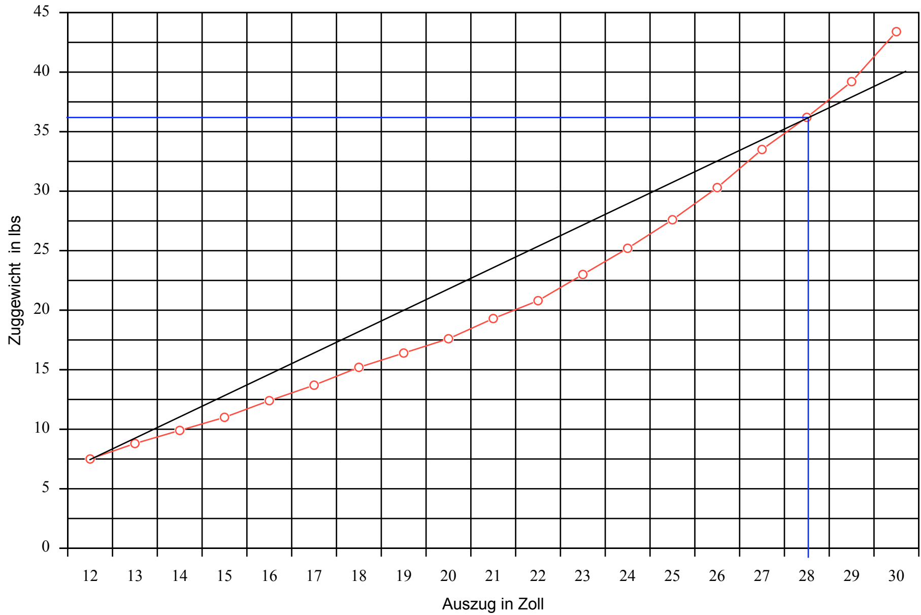
Auszugsdiagramm Horsebow 35#/28"
