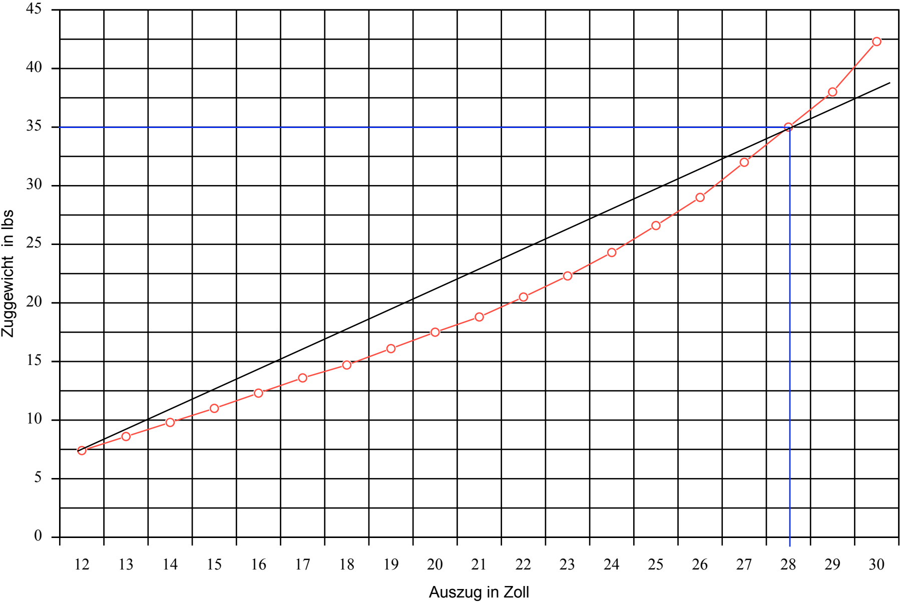
Auszugsdiagramm Horsebow Express 35#/28"
