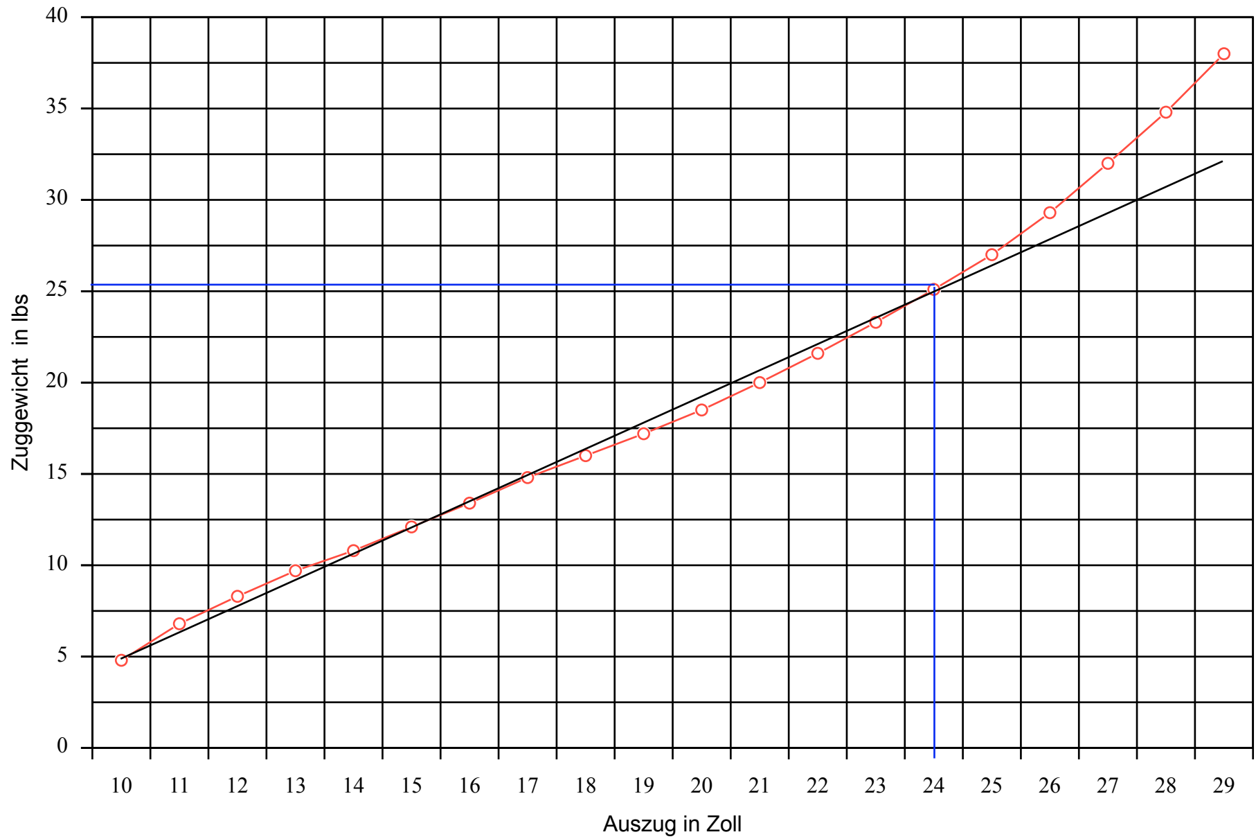
Auszugsdiagramm Mingo 48" 25#/24"
