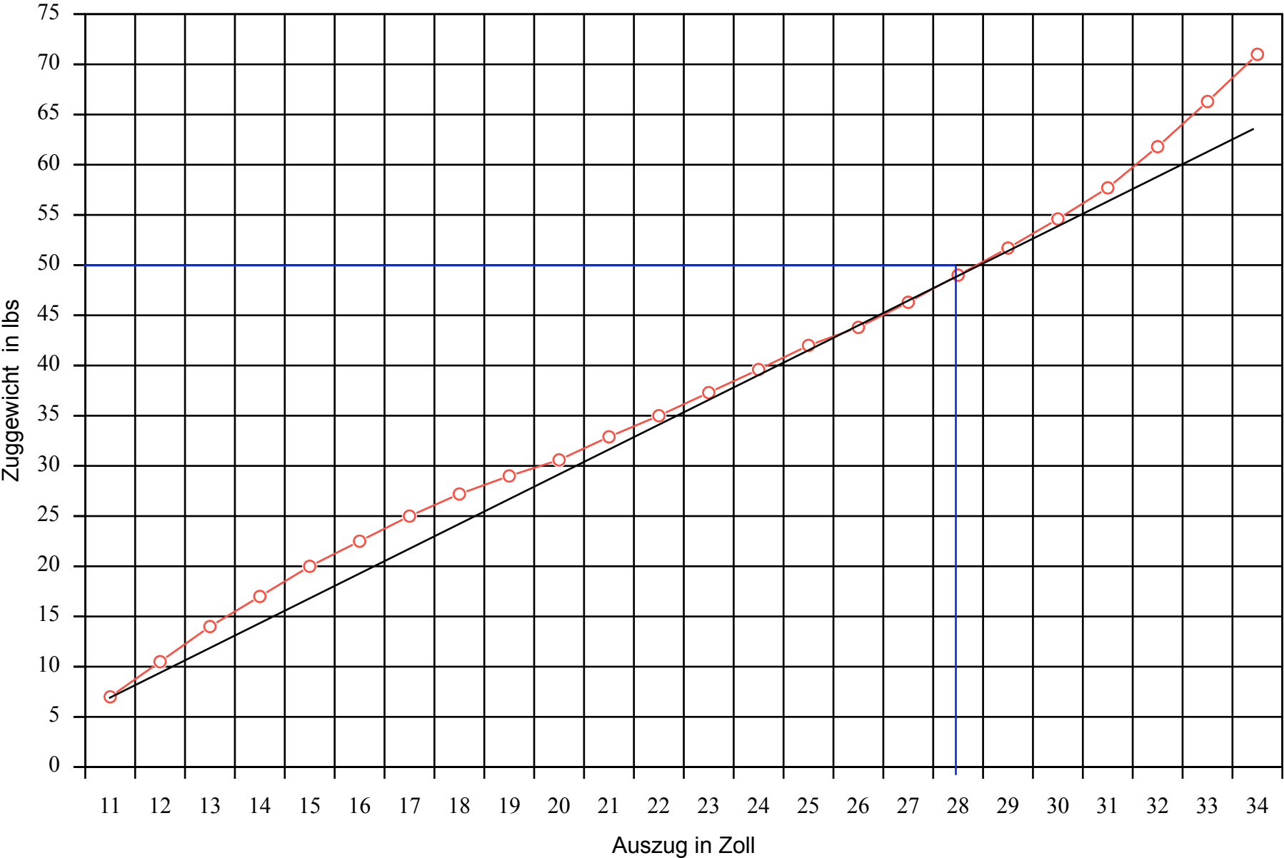
Auszugsdiagramm Quick Stick 60", 50#/28"
