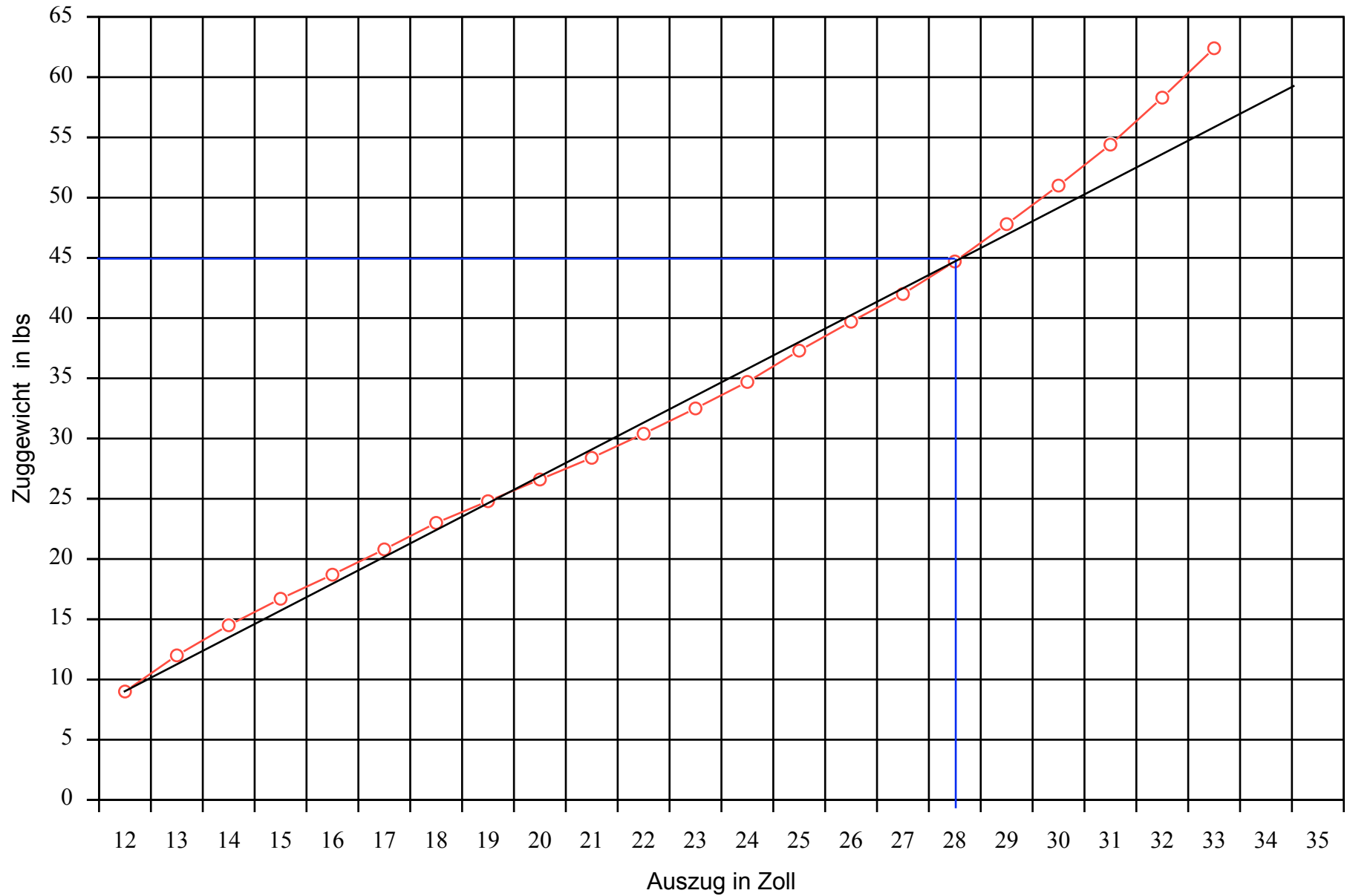
Auszugsdiagramm Raven 64", 45#/28"
