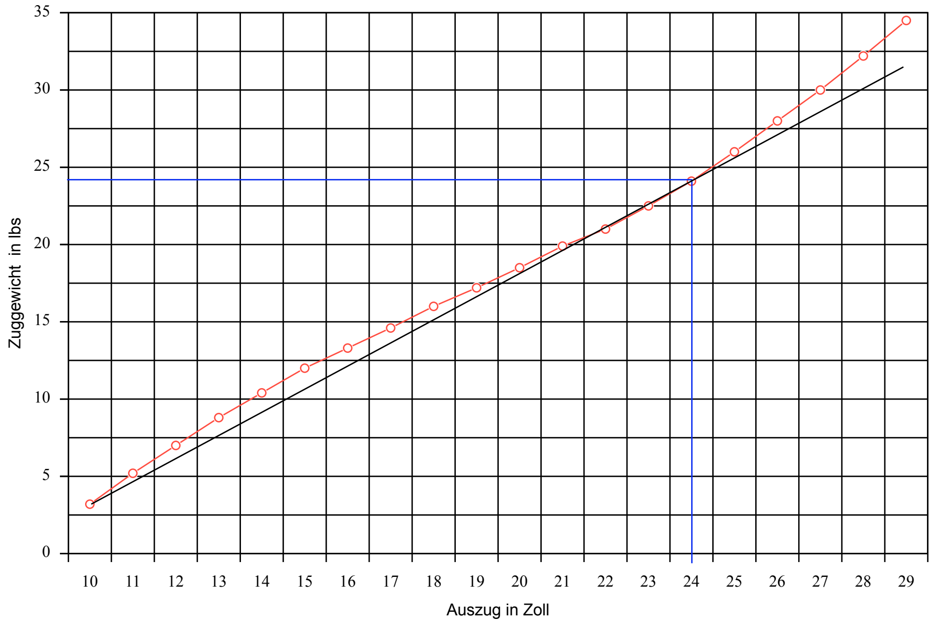
Auszugsdiagramm Tombow 50" 25#/24"
