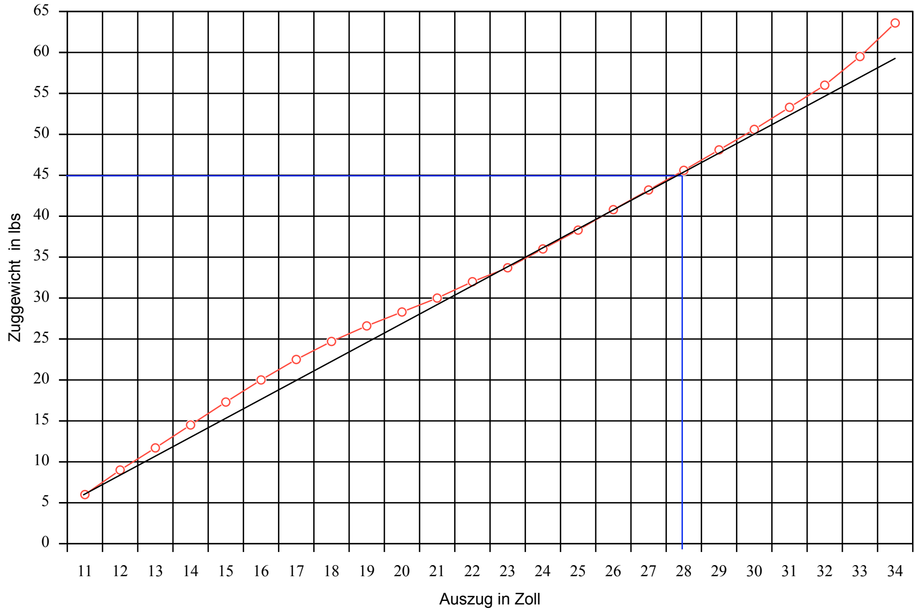
Auszugsdiagramm Viper 68", 45#/28"
